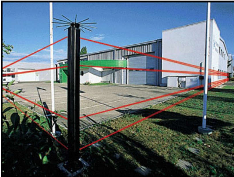
Barrière infrarouge extérieur de protection entrepot , site isolé
